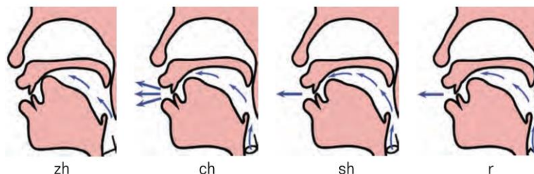
Рис. 2 Китайские шипящие
